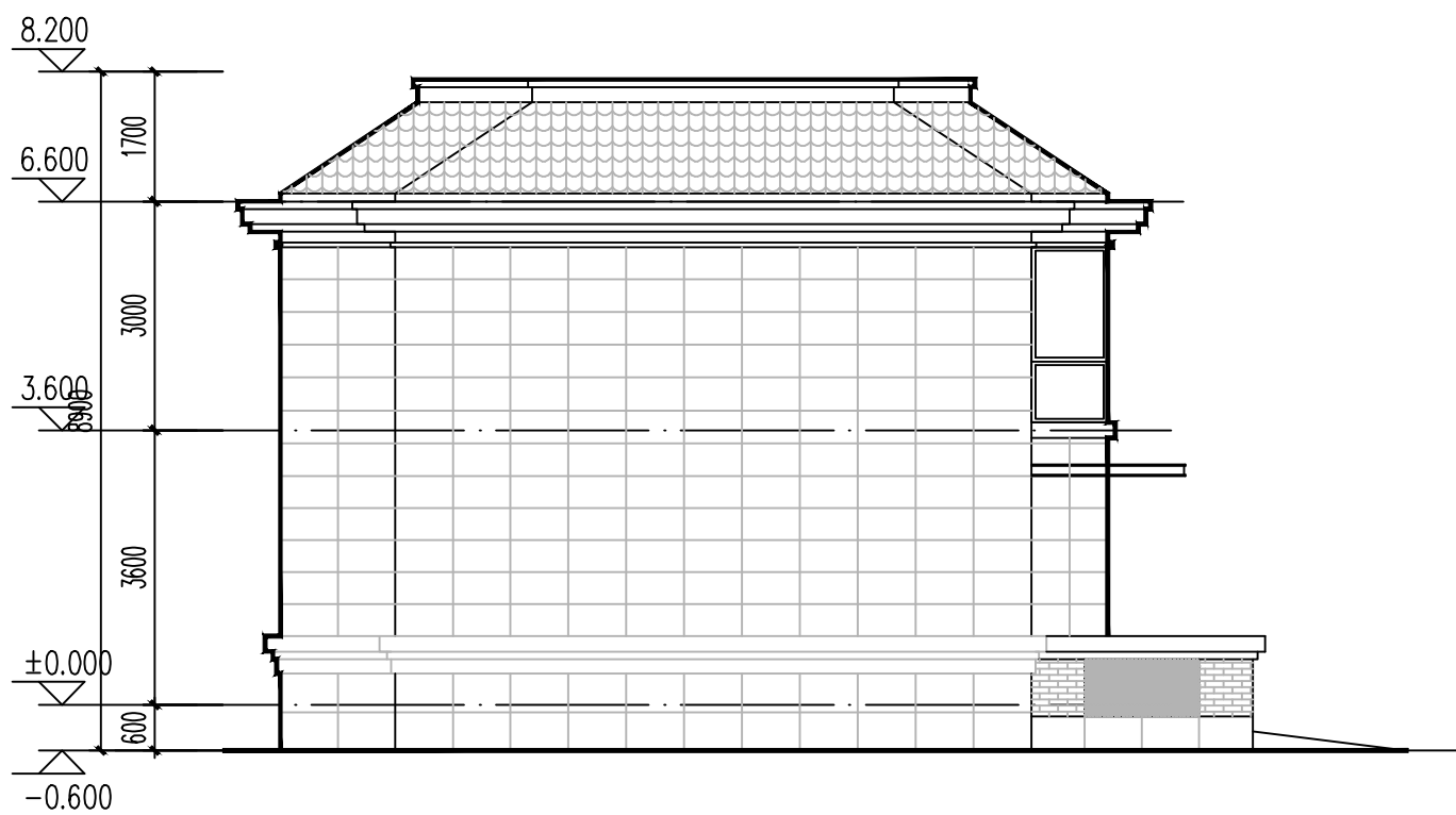
西立面图 1:100
