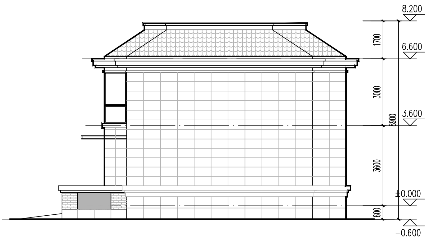
东立面图 1:100
